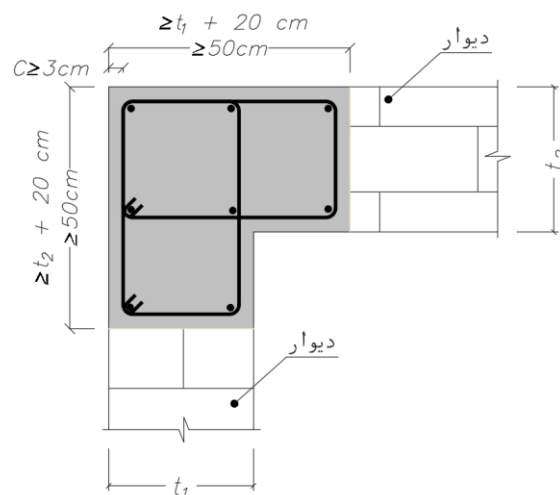
شکل ۸۴) حداقل ابعاد کلاف دوبل
