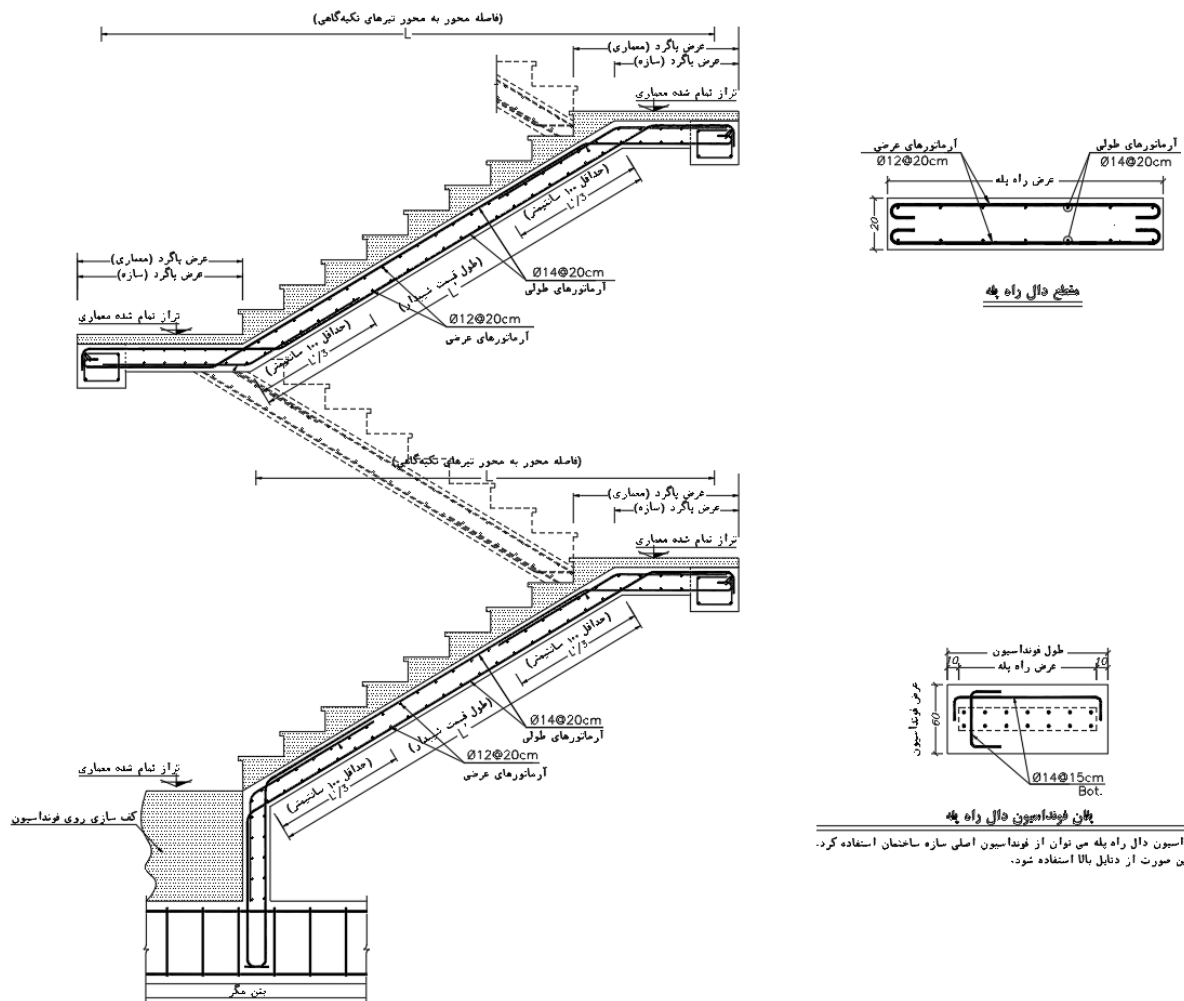
شکل ۱۰۴ جزئیات سازه ای پله بتنی
