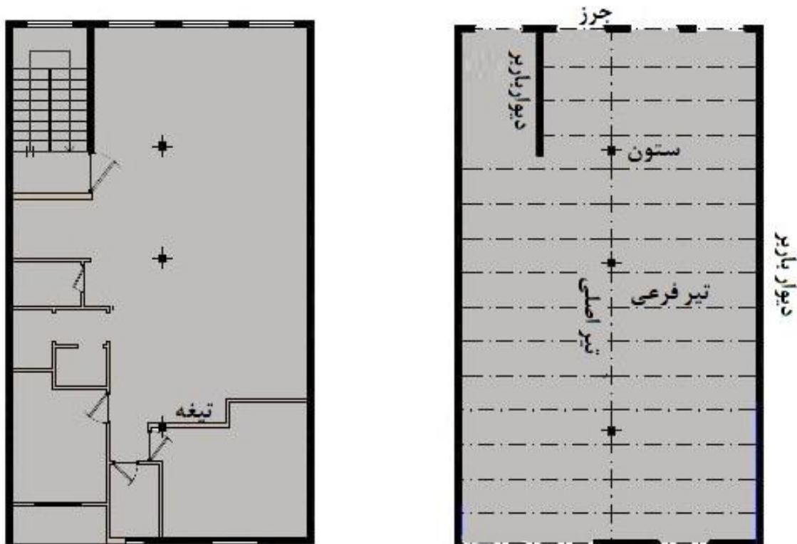
شکل ۵۴) آرایش دیوارها در یک امتداد (غیرمجاز)
