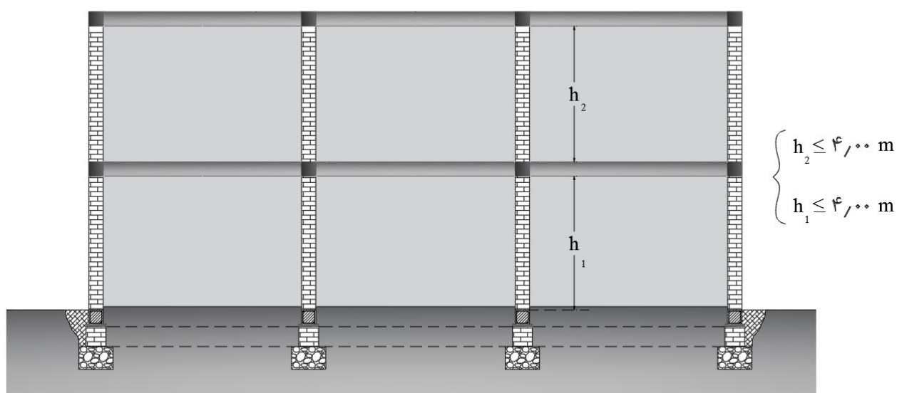
شکل ۹) حداکثر ارتفاع هر طبقه (از روی کلاف زیرین هر طبقه تا زیر سقف)
