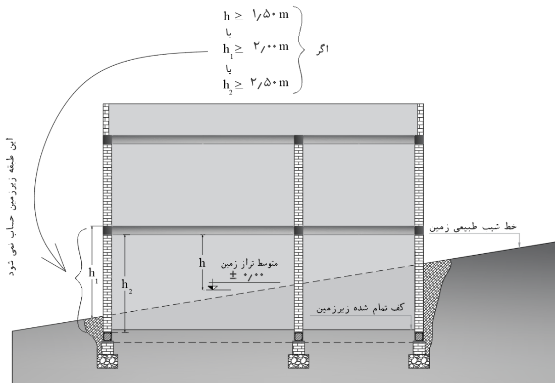
شکل ۸) محسوب نشدن یک طبقه به عنوان زیرزمین با توجه به تراز ارتفاع و ترازهای ارتفاعی آن - محدود بودن تعداد کل طبقات به دو طبقه با احتساب زیرزمین
